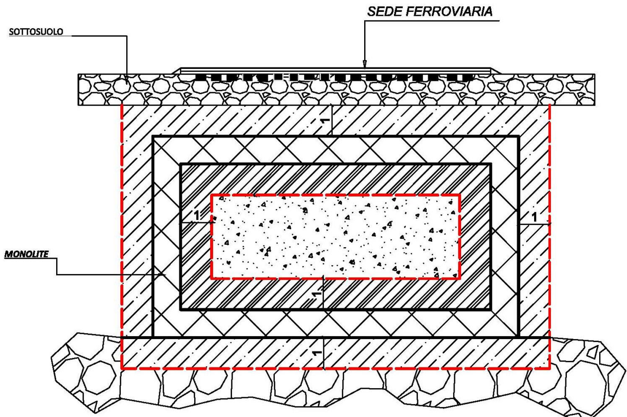
2. SEZIONE TRASVERSALE MONOLITE
