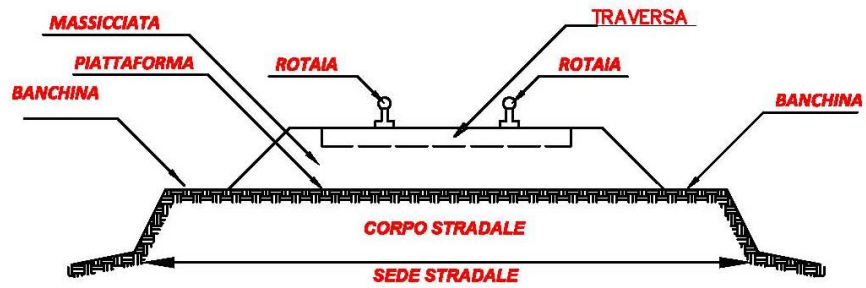
1. SEZIONE TRASVERSALE SEDE FERROVIARIA
